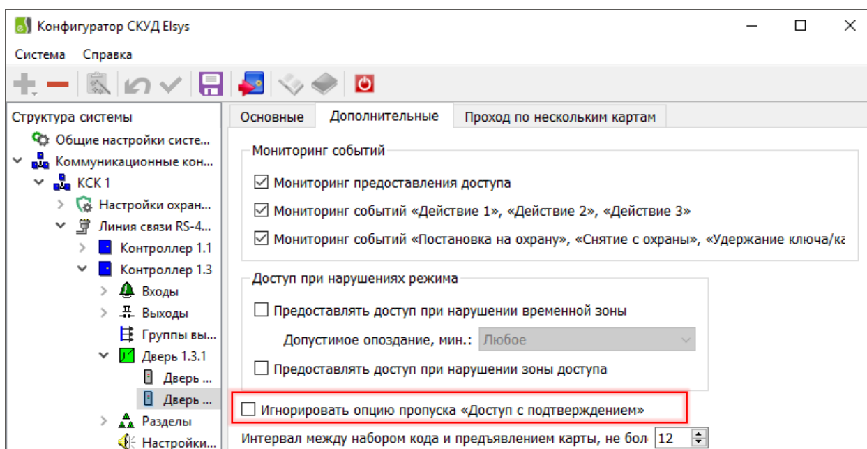
Рис. 31. Настройки считывателя, где необходимо выключить режимы «Доступ с подтверждением картой» и «Доступ с подтверждением кнопкой»
