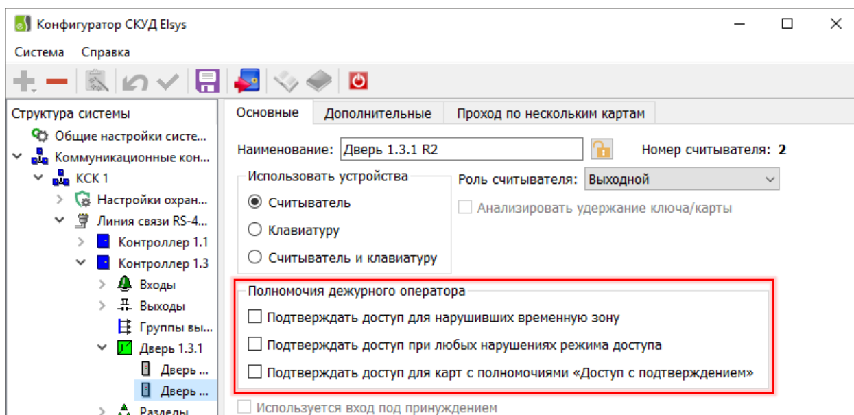
Рис. 34. Настройки считывателя, где используется режим «Доступ с подтверждением кнопкой»
