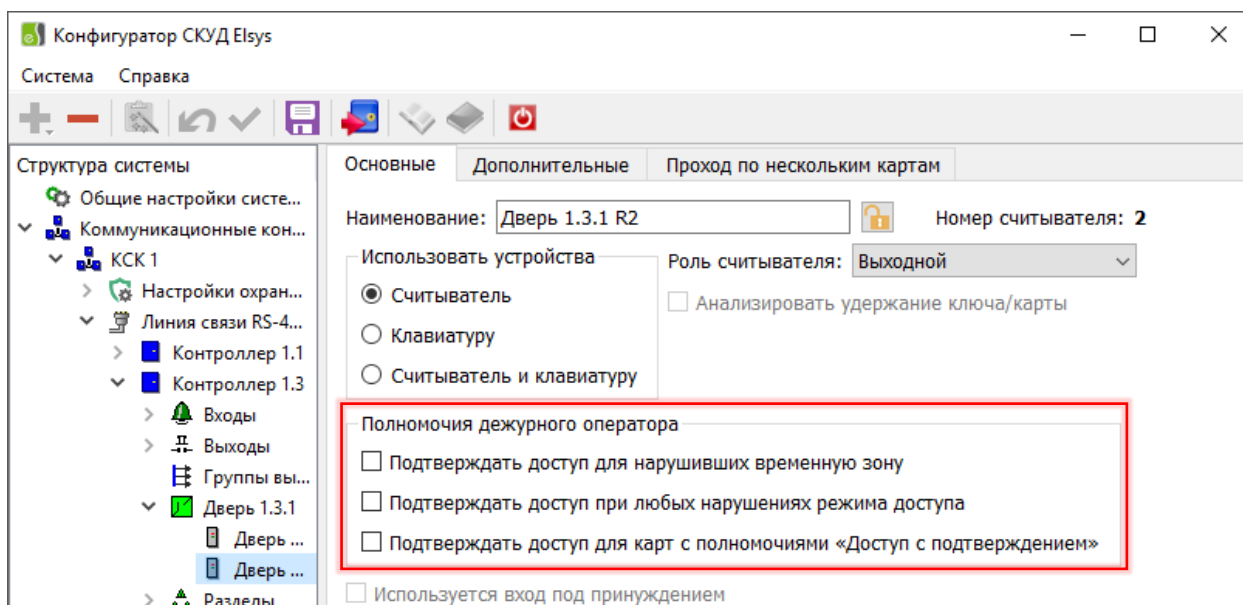
Рис. 30. Настройки считывателя, где используется режим «Доступ с подтверждением картой»
